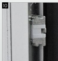
10 Zasuwница GU rygłowanie dolne
