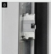
8 Zasuwница GU rygłowanie górne
