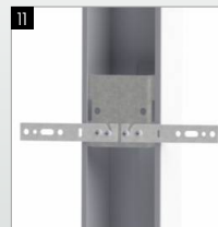
Elementy wzmacniające konstrukcję ościeżnicy z kotwami montażowymi
